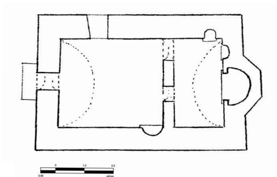
Κάτοψη Προφήτη Ηλία «Μετόχι» Πάρνηθας. Προσωρινή αποτύπωση, 25/01/2004. Ε. Κ. Παπαδοπούλου.
