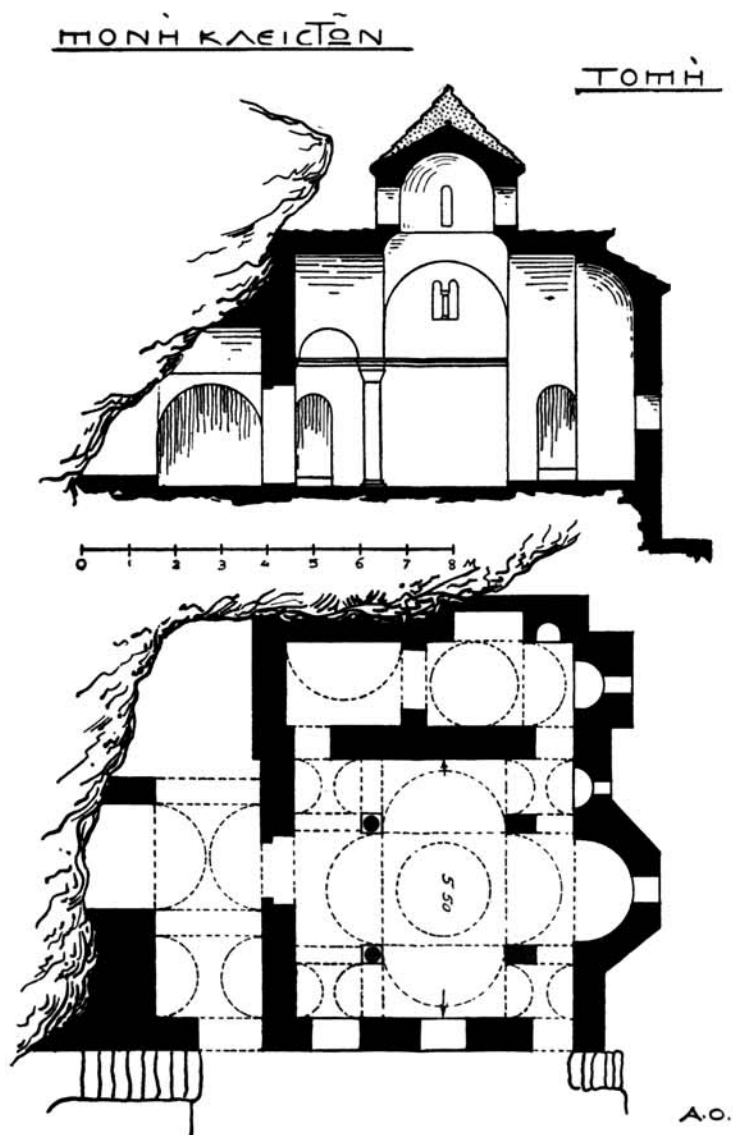
Κάτοψη και τομή του καθολικού της Ι. Μονής Κλειστών. Φωτο: Από το βιβλίο του Αναστ. Ορλάνδου (1933).
