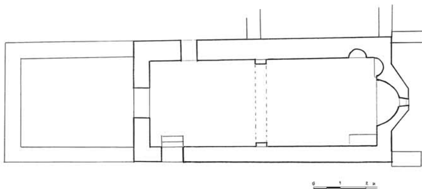
Άγ. Νικόλαος - Μετόχι Πάρνηθας. Προσωρινή αποτύπωση, Ιανουάριος 2004. Ελίζα Παπαδοπούλου.
